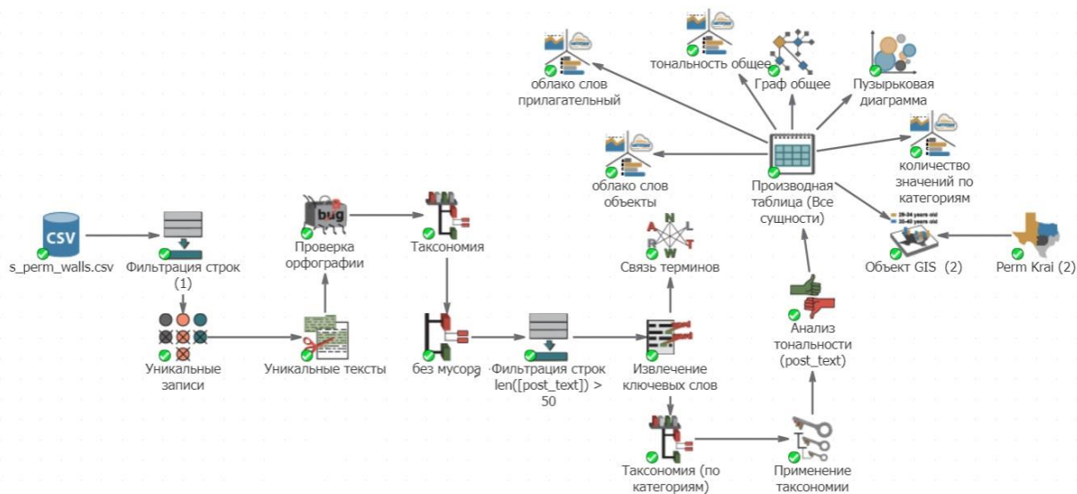
Рис. Общая схема анализа данных в PolyAnalyst
